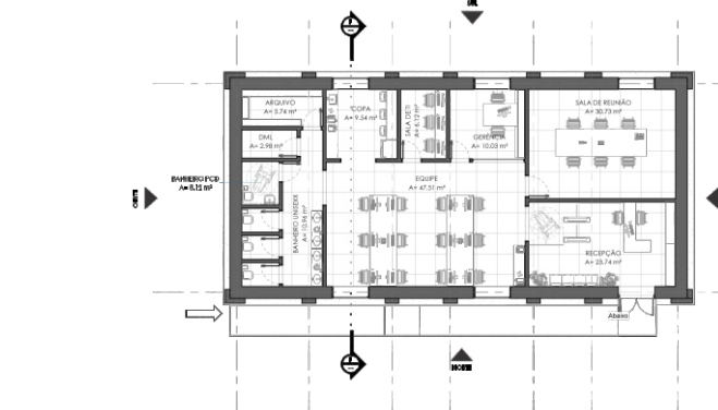
Administrativo - Galpão SPR
