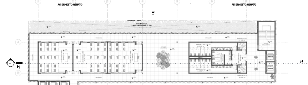
3 Pavimento - Estação Saber
