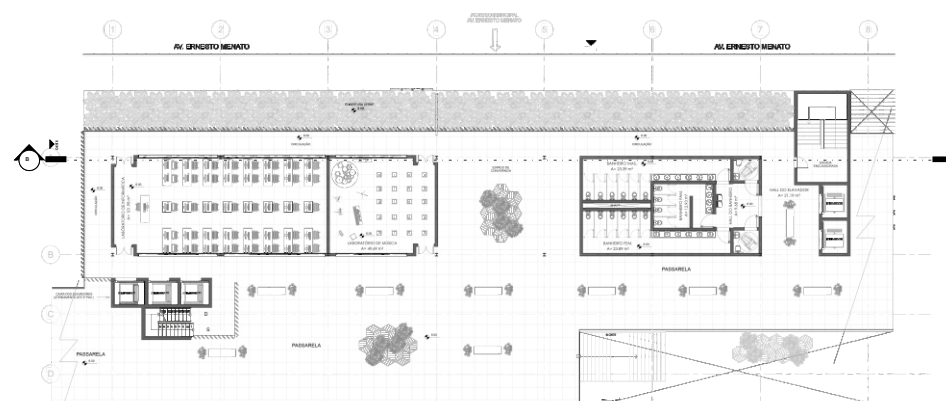
2 Pavimento - Estação Saber
