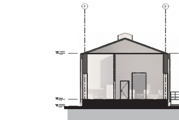
Corte Galpão SPR - Setor Adm.
