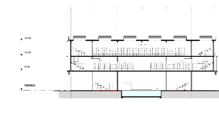
Corte Est. Movimento
