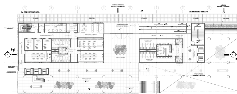
1 Pavimento - Estação Saber
