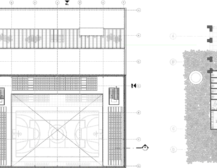
Mezanino - Auditório
