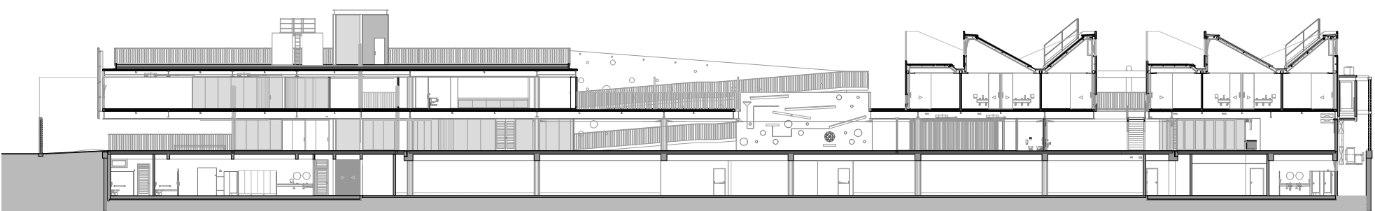
corte ee
