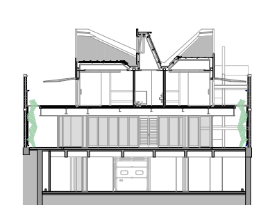
corte dd
