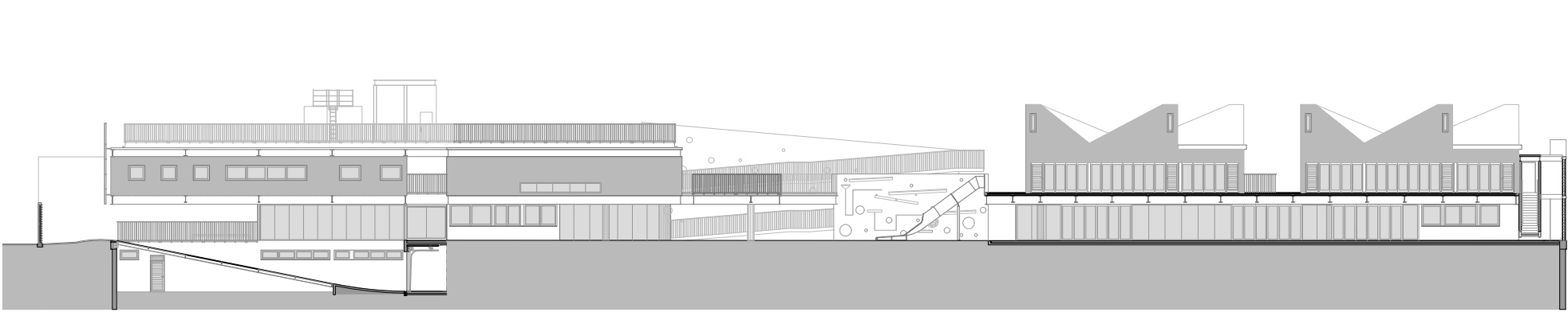
corte gg
