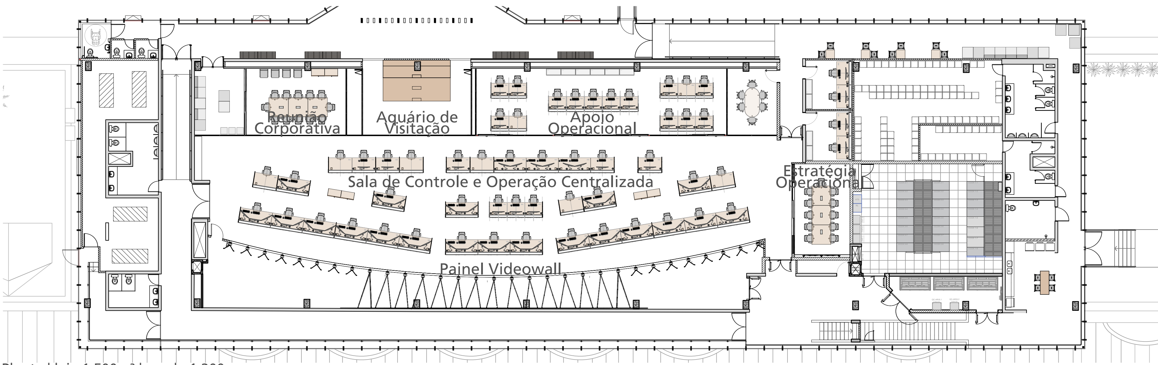
Planta | laje 1.500m² | escala 1:200
